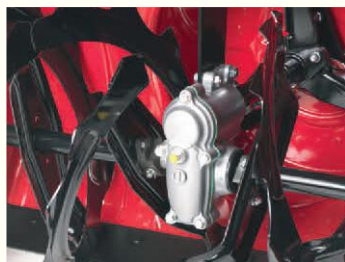
Automatische Schneckenabschaltung
