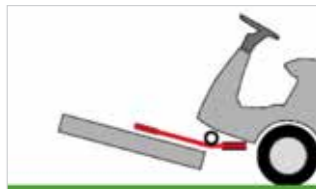
Zwei kugelgelagerte Führungsrollen gewährleisten das Fluchten des Keilriemens auch bei Geländeunebenheiten.
